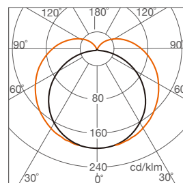
灯具配光曲线 (3000K, 4000K, 6500K)
