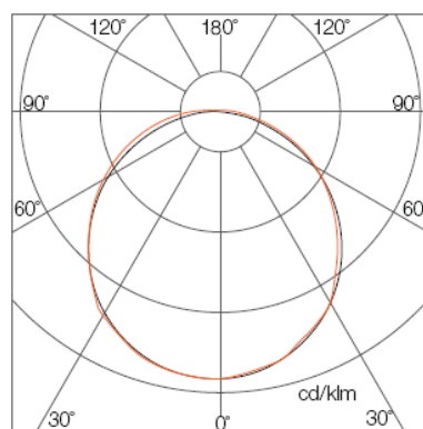
URG22 - 灯具配光曲线
