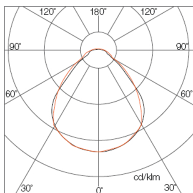
URG19 - 灯具配光曲线
