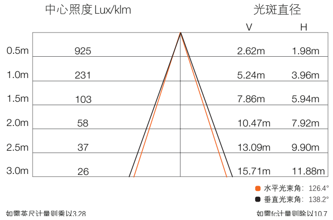
照度分布
